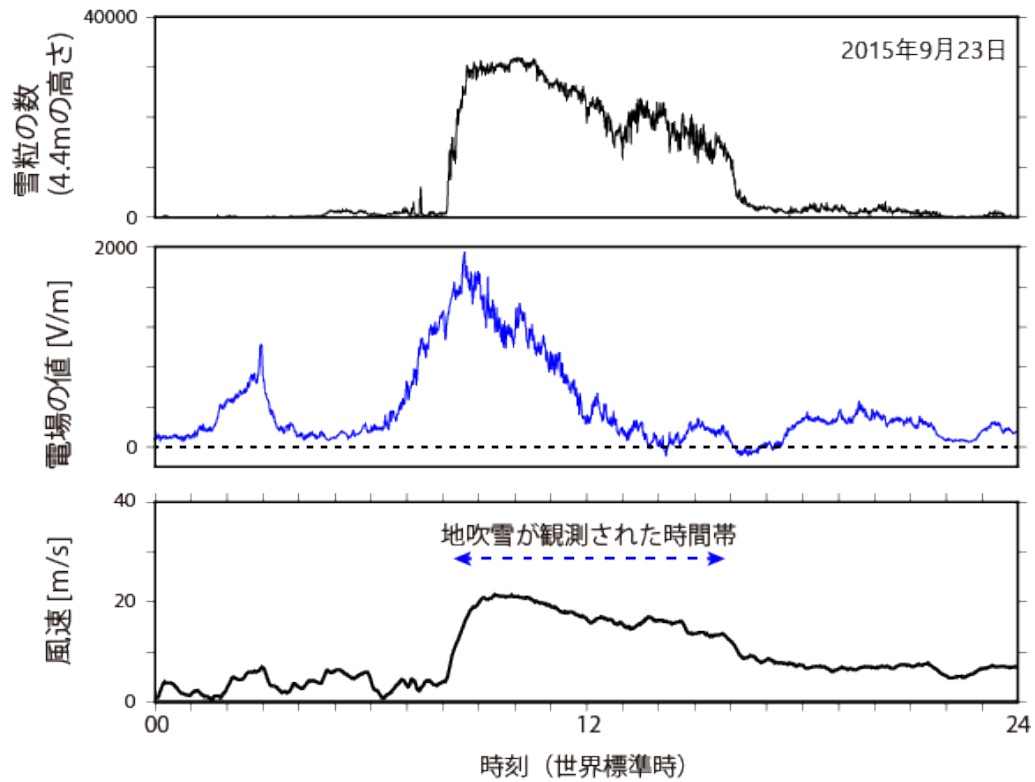
図1 2015年9月23日の雪粒の数、電場の観測値、風速の推移
